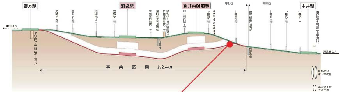
図1：連続立体交差予想縦断面図
