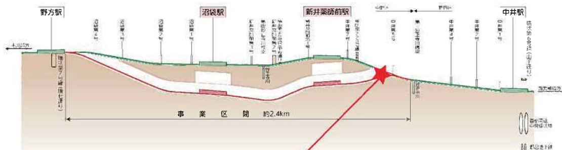
図1：連続立体交差予想縦断面
